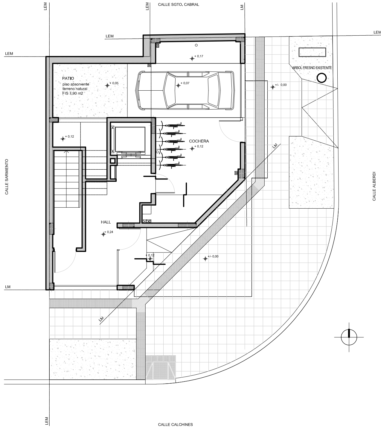
PLANTA BAJA TOTAL SUPERFICIE CUBIERTA: 89,50 m 2
